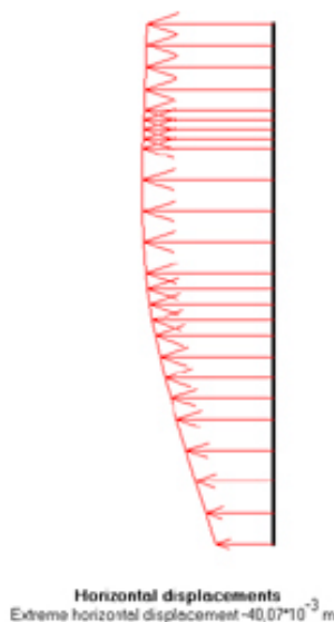
Σχήμα 4-4: Οριζόντιες μετακινήσεις διαφραγματικού τοίχου στη θέση A-1
